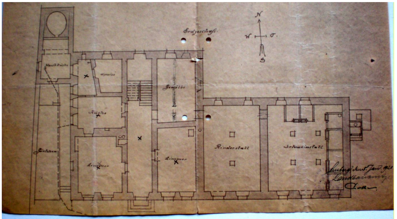
Erdgeschoss (unten) und Obergeschoss bis 1968
